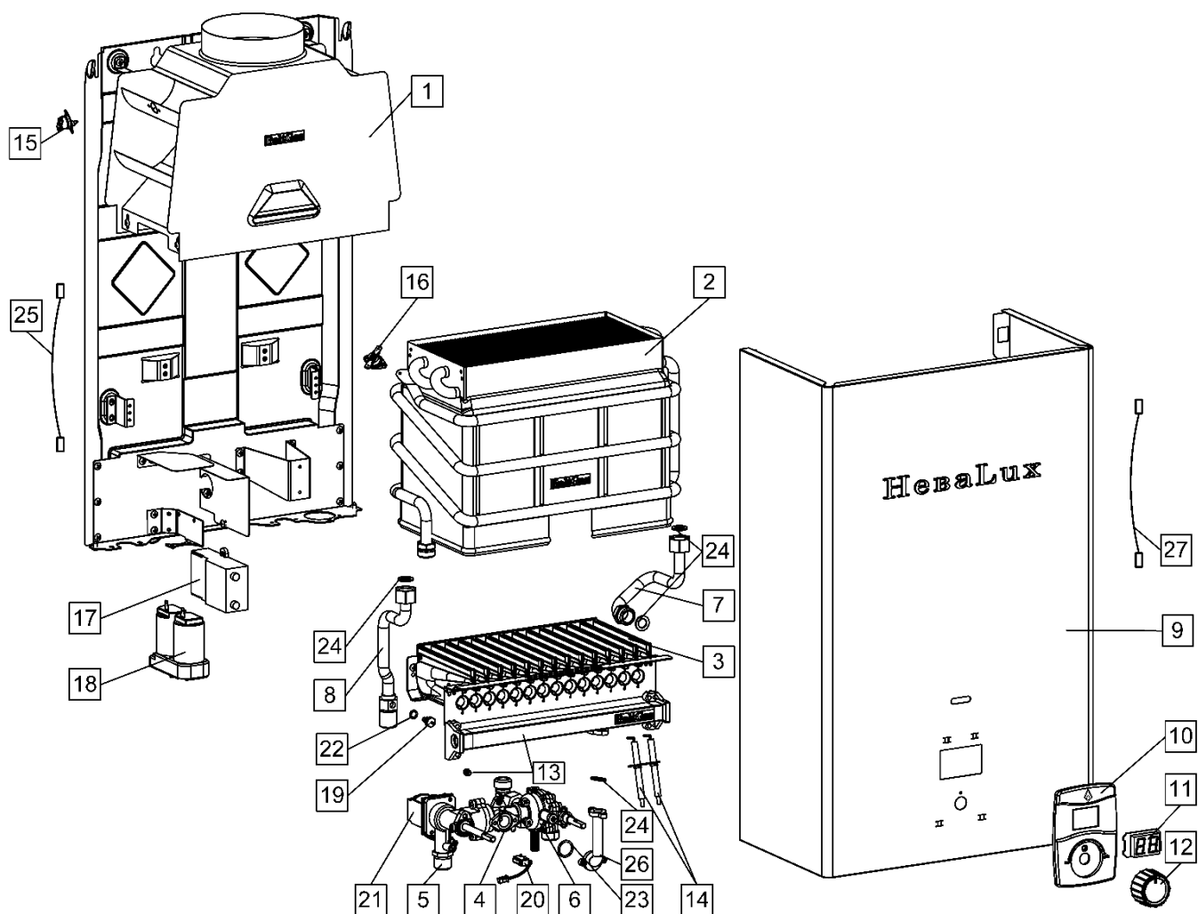
Рисунок 11а. Вид аппарата «НеваLux 5514» с разнесёнными частями
