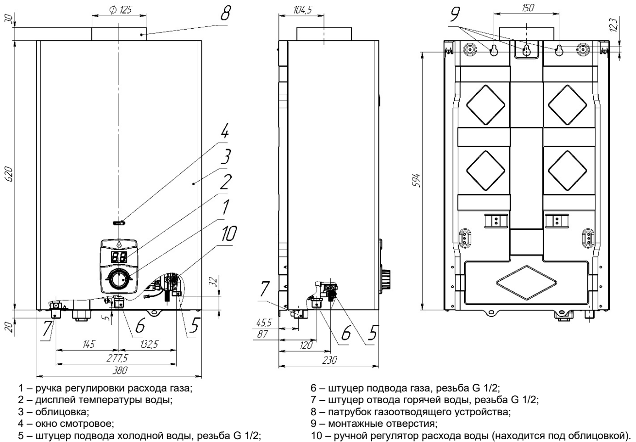
Рисунок 1а. Габаритные и присоединительные размеры аппарата «NevaLux 5514»
