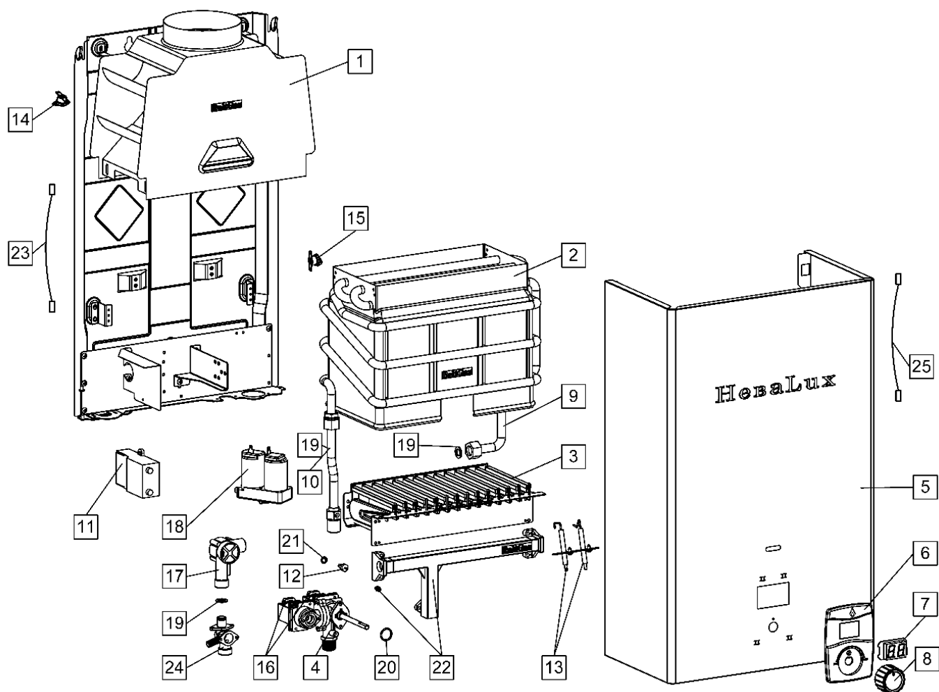
Рисунок 116. Вид аппарата «НеваLux 5514Е» с разнесёнными частями
