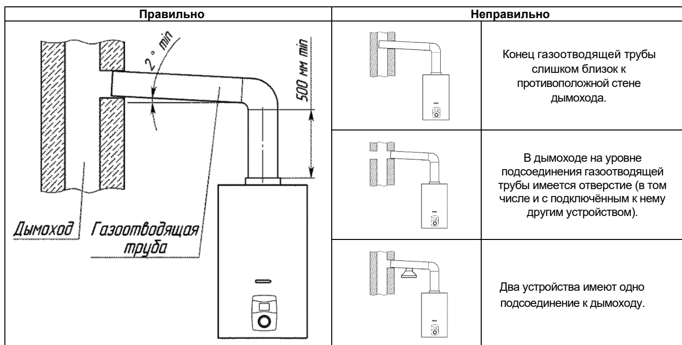
Рисунок 8. Подключение аппарата к дымоходу
