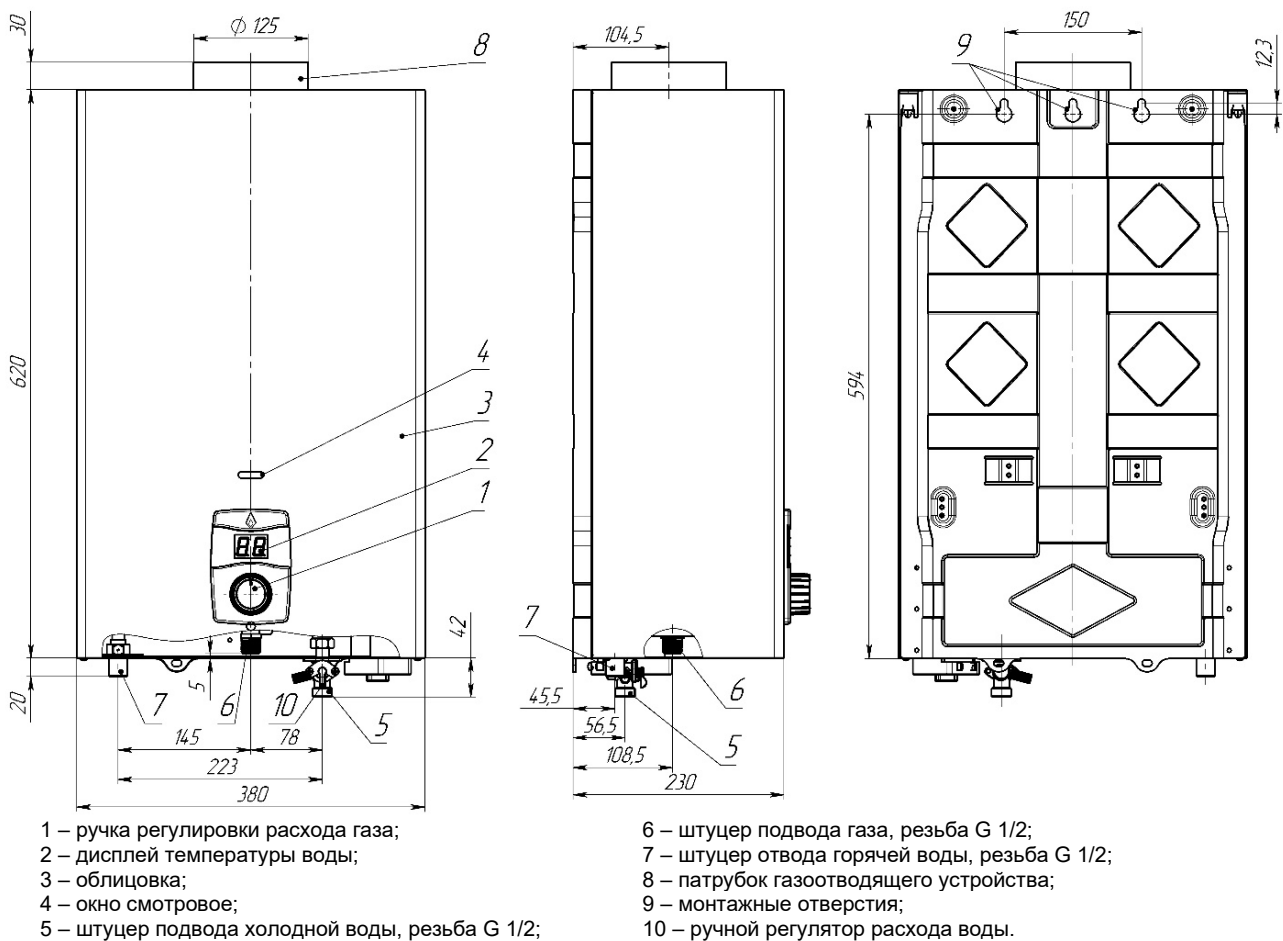
Рисунок 1б. Габаритные и присоединительные размеры аппарата «NevaLux 5514E»
